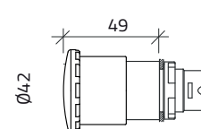
PULSANTIERE DI EMERGENZA 080CA0808-6GEAS
