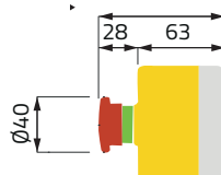
PULSANTIERE DI EMERGENZA 080CA0808-6GA
