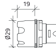
SELETTORE 4 POSIZIONI INSERTO BIANCO
