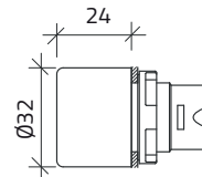
SELETTORE 3 POSIZIONI INSERTO BIANCO
