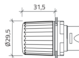
UNITA' ALTA CON GEMMA LUMINOSA
