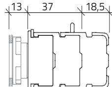
SISTEMI DI PROTEZIONE (CAPPUCCIO IN GOMMA PULSANTI DOPPI)
