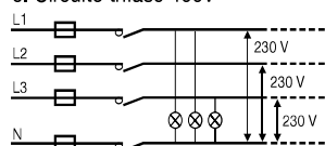
c. Circuito trifase 400V
